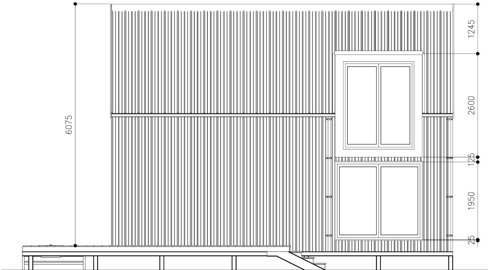
ELEVATION 02
