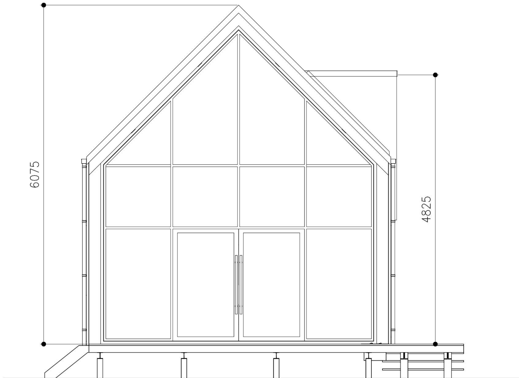
ELEVATION 01
